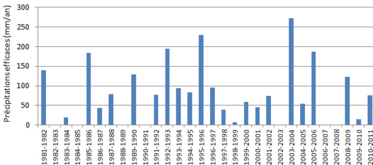
Figure 15 : Précipitations efficaces des 30 dernières années (station météo de Perpignan)
